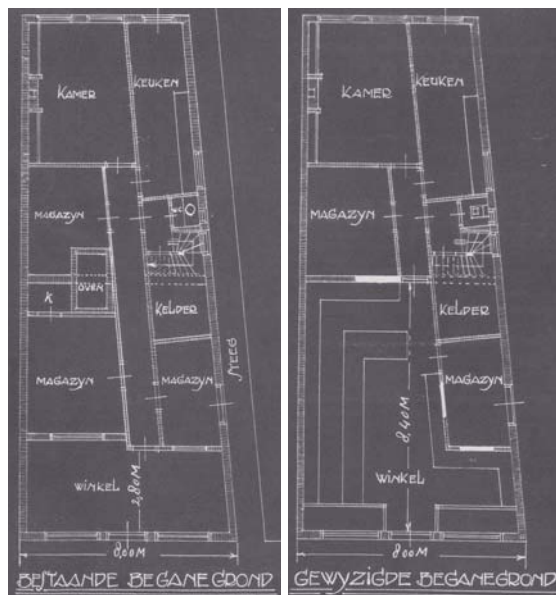
Bouwtekening uit 1928 van oude en nieuwe situatie begane grond.
